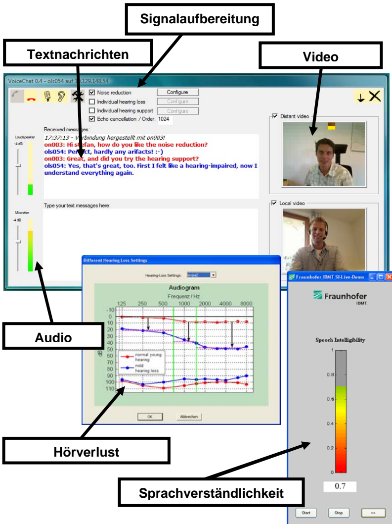
Abbildung 6: Das entwickelte Kommunikationssystem beinhaltet Signalaufbereitung, personalisierte Signalverstärkung sowie eine automatische Überwachung der Sprachverständlichkeit.
