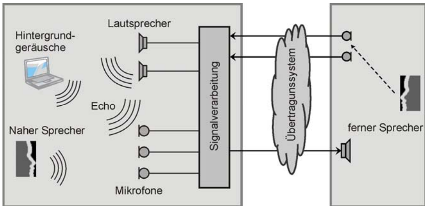
Abbildung 1: Problematik bei akustischen Kommunikationssystemen. Das Sprachsignal des nahen Sprechers wird überlagert von Hintergrundgeräuschen, Echos und Nachhall sowie dem empfangenen Signal des fernen Sprechers.
