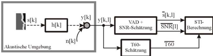
Abbildung 4: Schematische Darstellung des Verfahrens zur kontinuierlichen Berechnung des STI aus einem Mikrofonsignal, das Sprache, Rauschen und Verhallung enthält. Die zur Berechnung des STI notwendigen Parameter Signal-zu-Rauschabstand (signal-to-noise ratio, SNR) und Nachhallzeit des Raumes (T60) werden dazu blockweise geschätzt.
